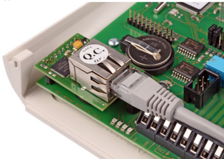
Obr. 14: nasazený modul převodníku Ethernet – GIPort
